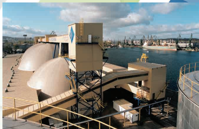
Bałtycka Baza Masowa, Zakłady Azotowe „Puławy” S.A.
