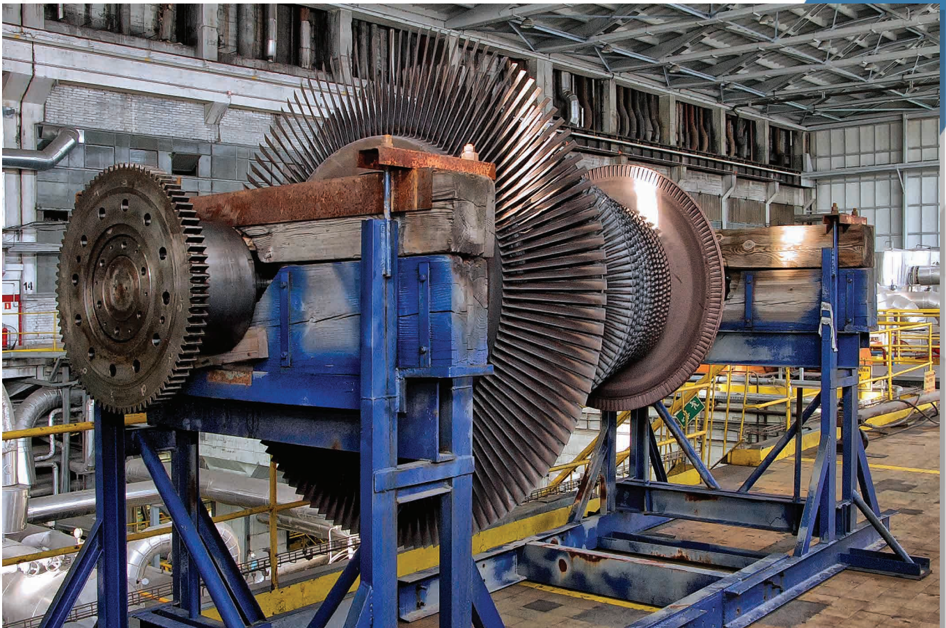
Demontaż turbozespołu TG2 dla Zakładów Azotowych „Puławy” S.A.
