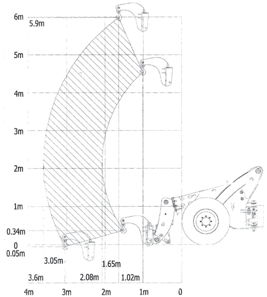
PODNOŚNIK TELESKOPOWY HT 285 udźwig 2,8t wysięg 6m
