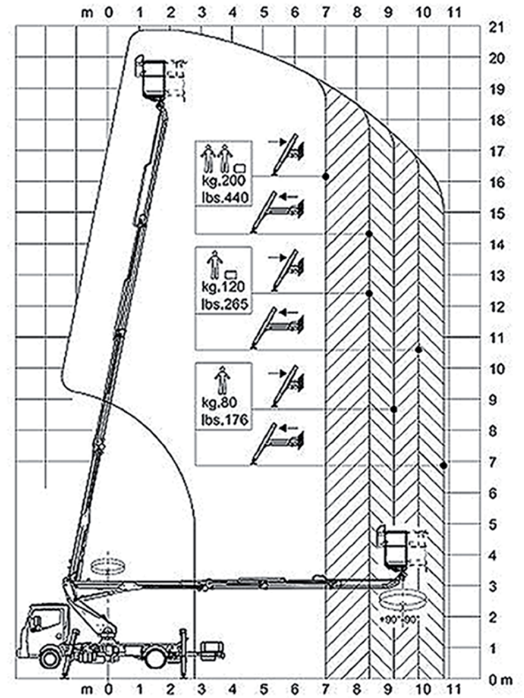
PODNOŚNIK KOSZOWY NISSAN GT 21-10 udźwig 200kg wysokość robocza 21m
